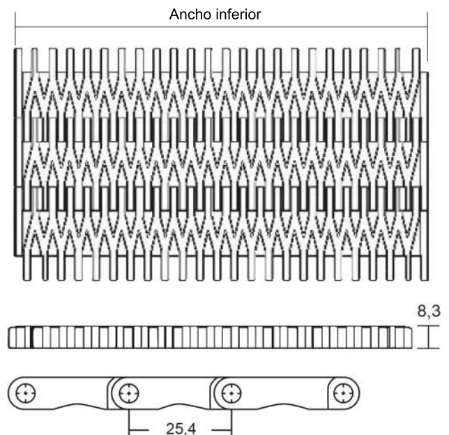
Dibujo técnico:
